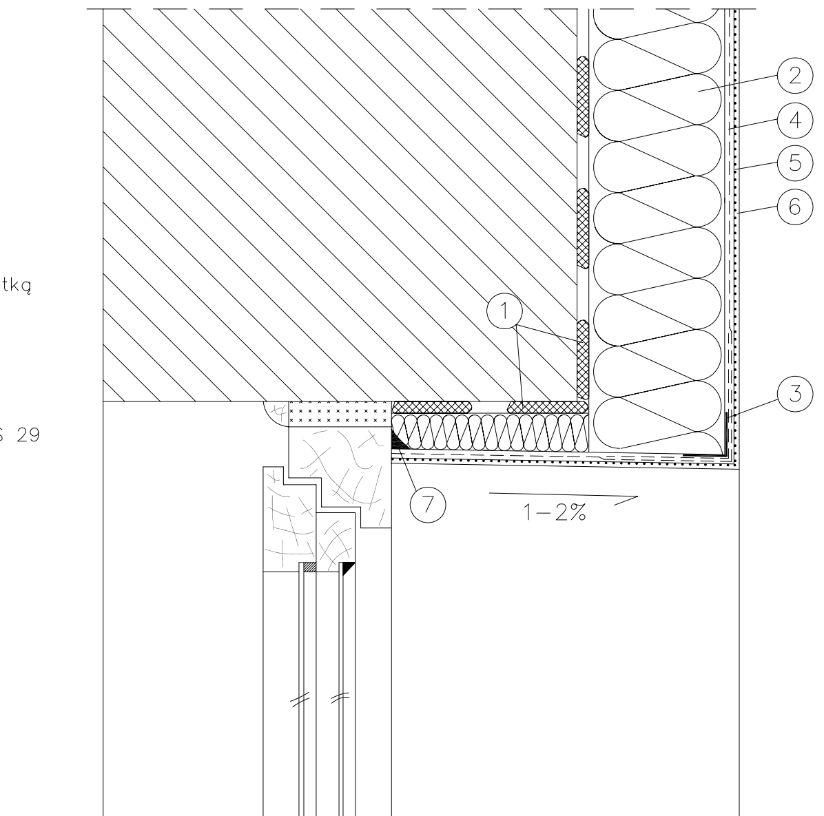
Rys. 7.16 Docieplenie nadproża
