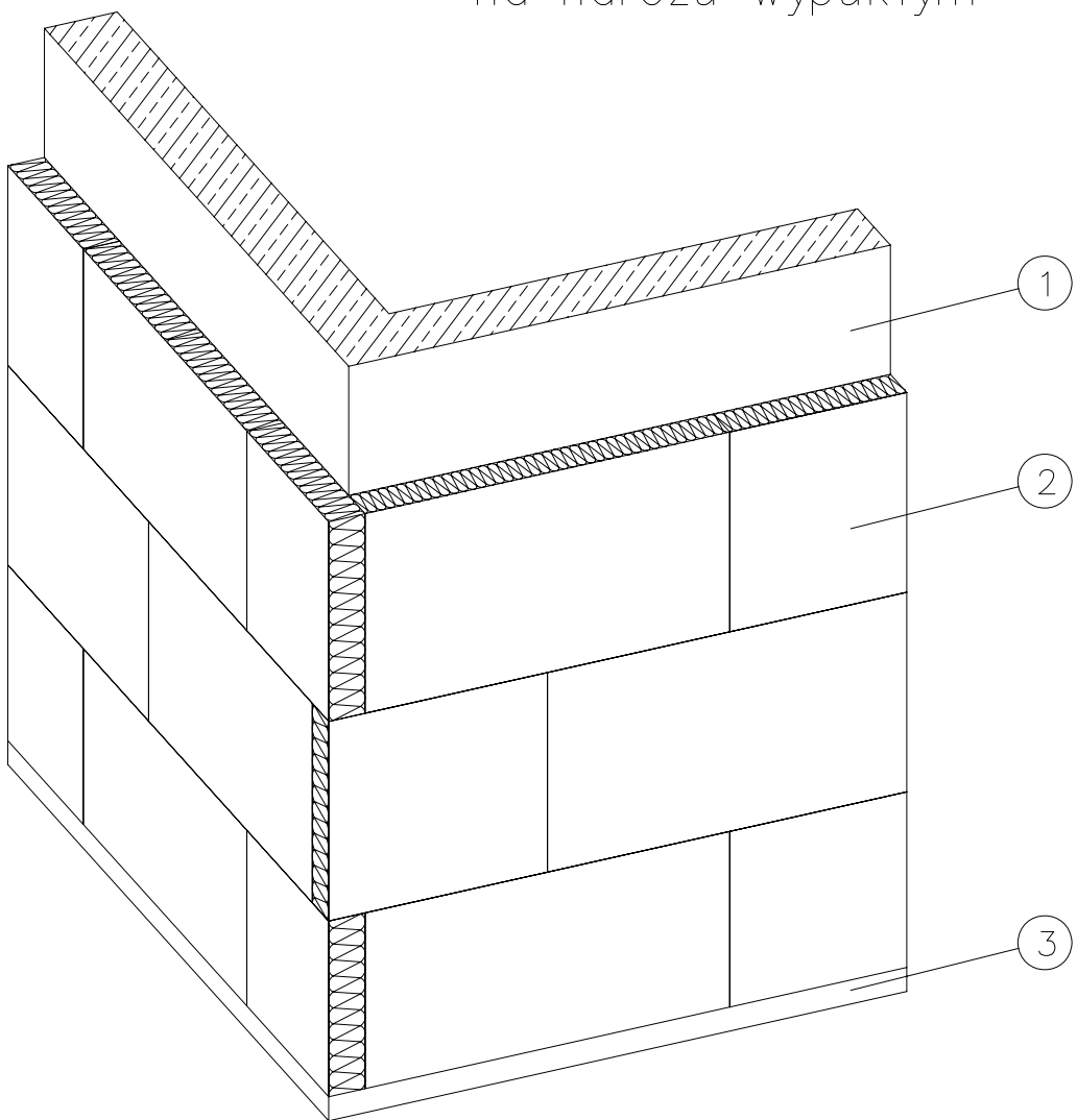
Rys. 7.1 Układ płyt termoizolacyjnych na narożu wypukłym
